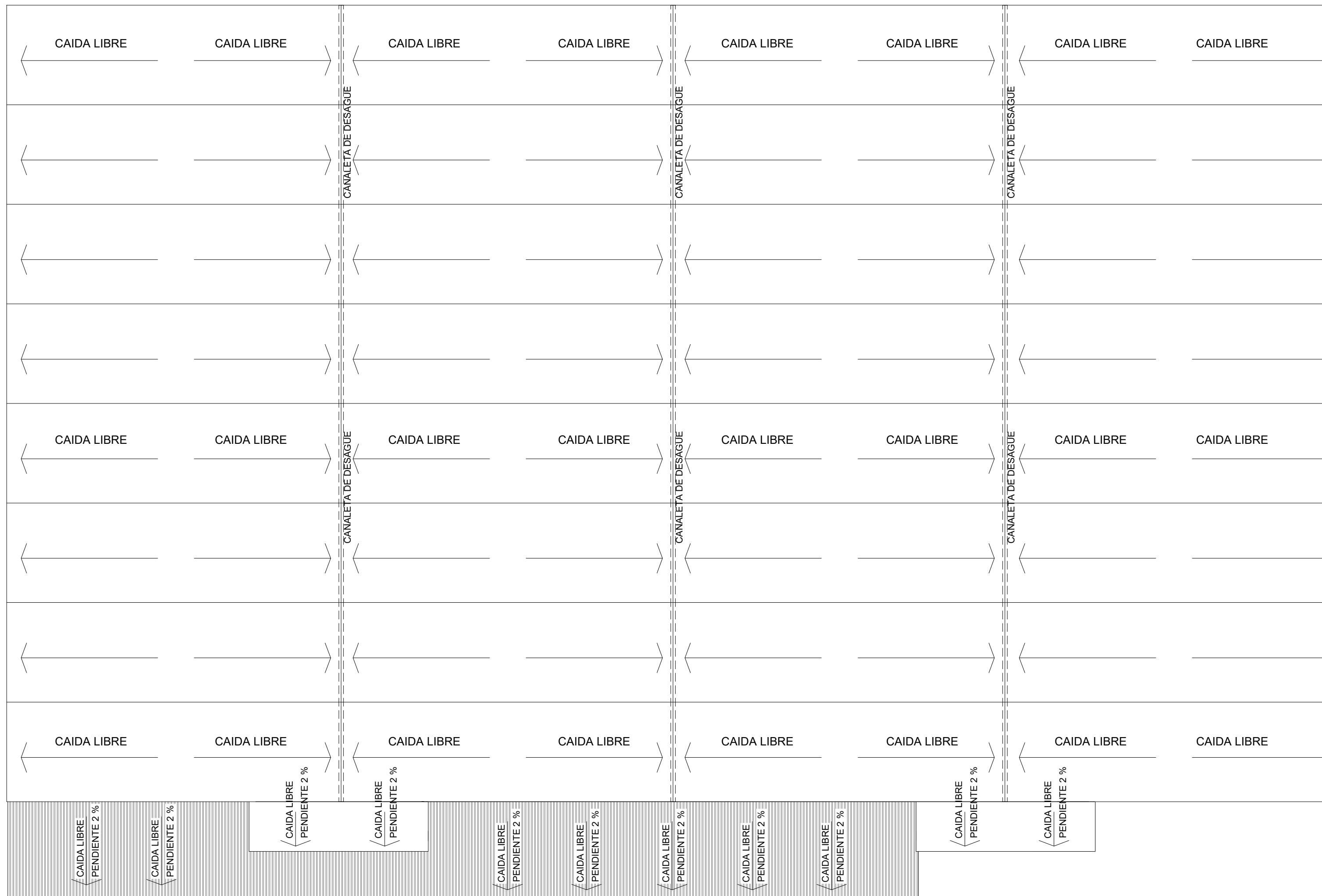
PLANTA DE TECHOS ESC. 1:100
